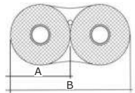
DN20: A:55 mm, B: 110 mm
